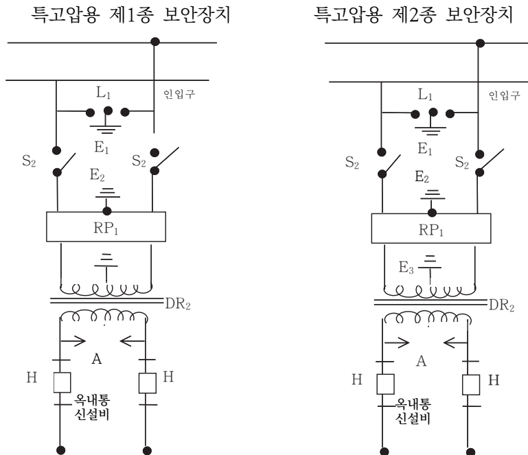
그림 362.5-4 고압용 제1종 및 제2종 보안장치
