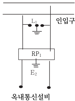
그림 362.5-1 급전전용통신선용 보안장치
