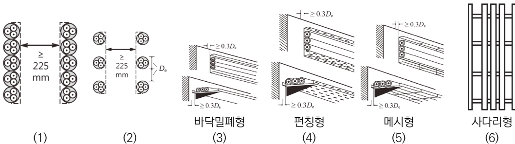
그림 232.41-3 수직트레이의 다심케이블 공사방법
