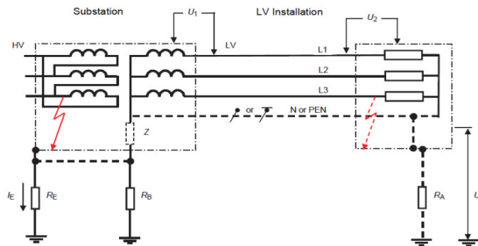
그림 213.1-1 고압계통의 지락고장 시 저압계통에서의 과전압 발생도
