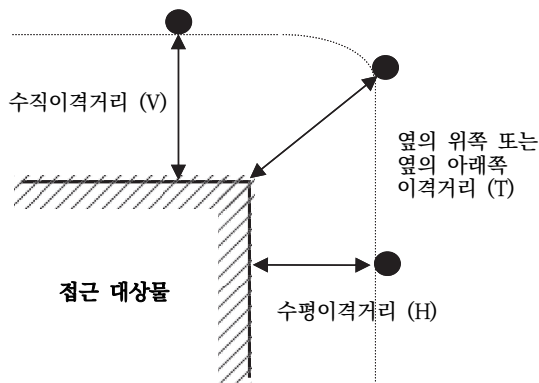
그림 332.11-1 이격거리의 관계
