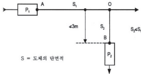
그림 212.5-1 분기회로 단락보호장치( P_2 )의 제한된 위치 변경
