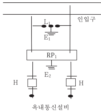
그림 362.5-2 저압용 보안장치
