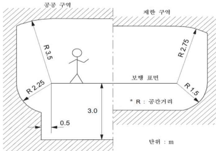
그림 461.1-2 공칭전압이 교류 1 kV 초과 25kV 이하인 경우 또는 직류 1.5 kV 초과 25 kV 이하인 경우 사람이 접근할 수 있는 보행표면의 공간거리
