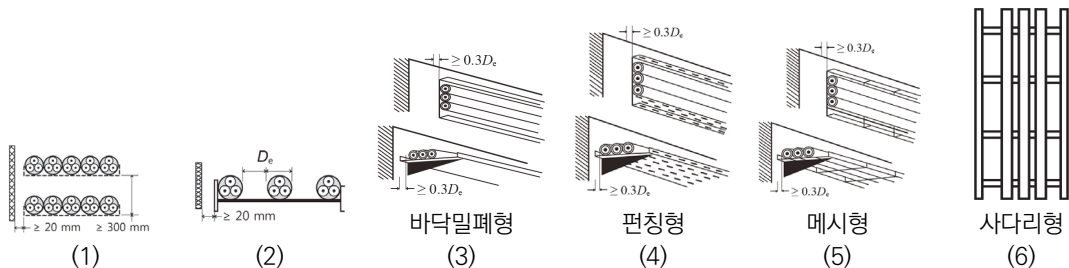
그림 232.41-1 수평트레이의 다심케이블 공사방법
