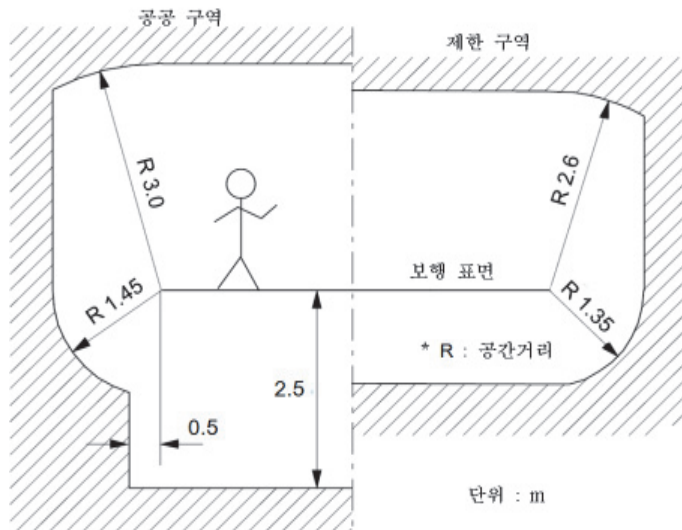
그림 461.1-1 공칭전압이 교류 1 kV 또는 직류 1.5 kV 이하인 경우 사람이 접근할 수 있는 보행표면의 공간거리
