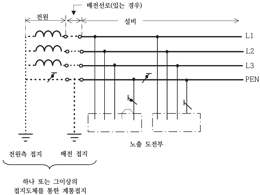
그림 203.2-4 TN-C 계통
