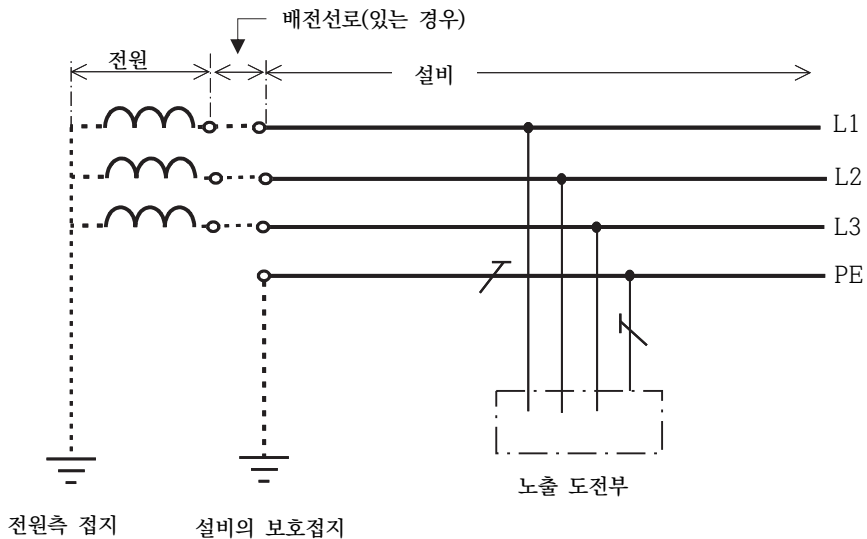
그림 203.3-2 설비 전체에서 접지된 보호도체가 있으나 배전용 중성선이 없는 TT 계통
