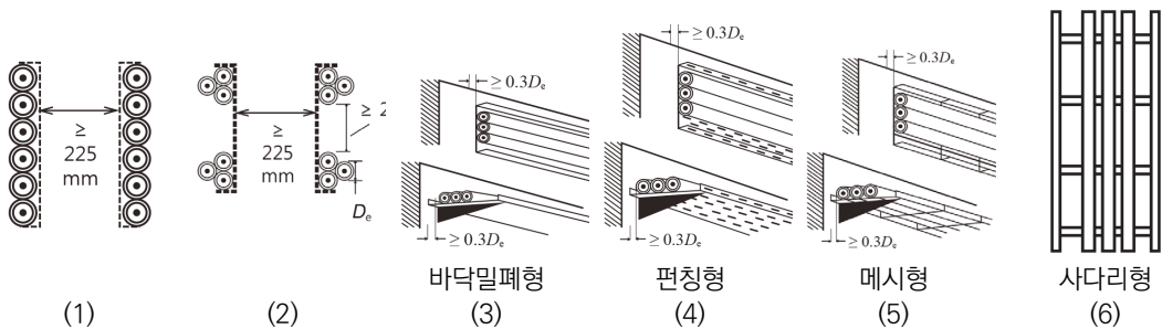
그림 232.41-4 수직트레이의 단심케이블 공사방법
