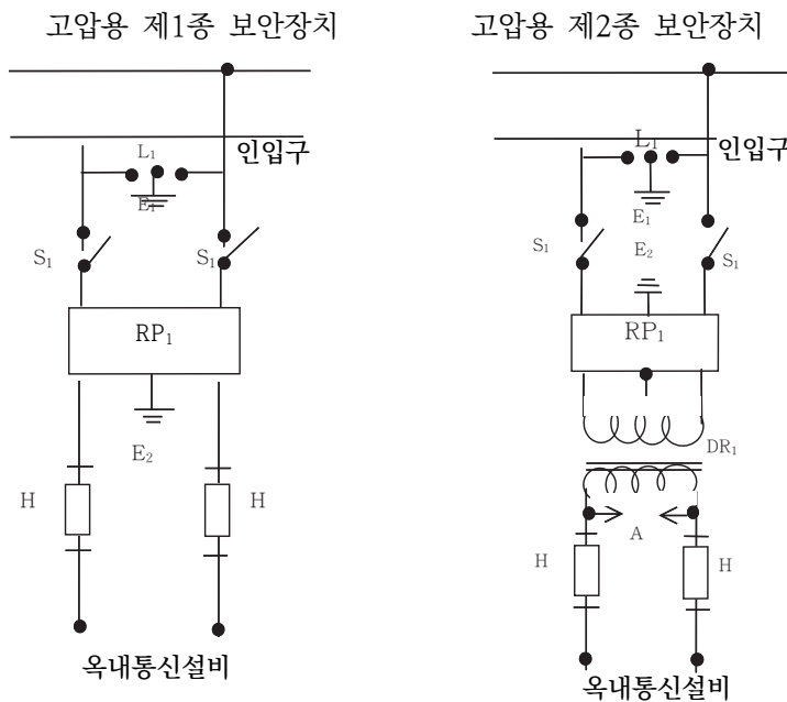
그림 362.5-3 고압용 제1종 및 제2종 보안장치
