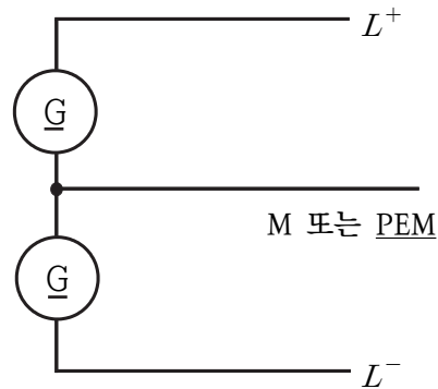
그림 202.1-2 3선식
