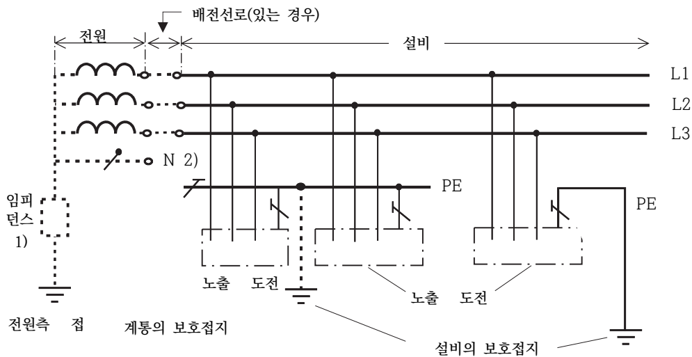
그림 203.4-2 노출도전부가 조합으로 또는 개별로 접지된 IT 계통
