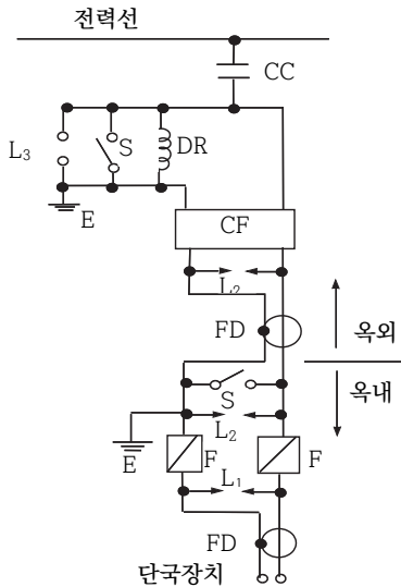
그림 362.10-1 전력선 반송 통신용 결합장치의 보안장치
